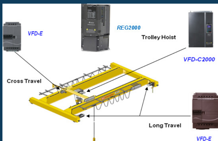
Biến tần cho cầu trục
